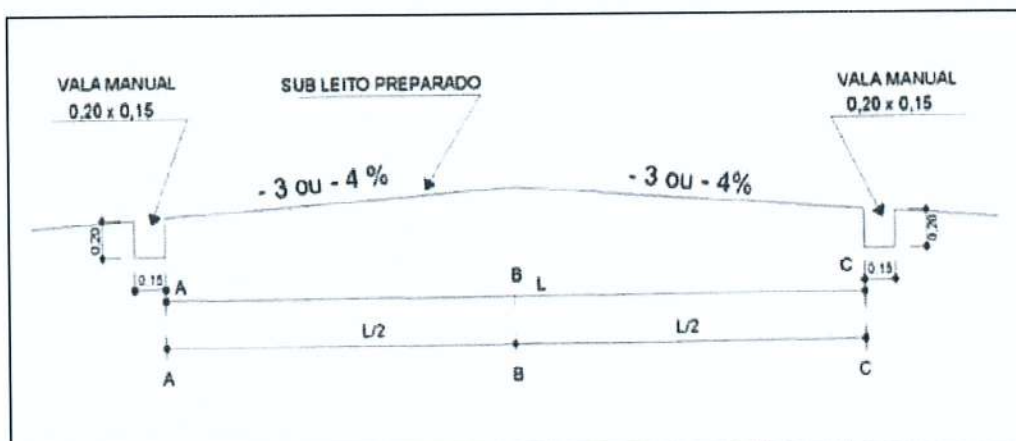
Figura 9: Valas Laterais
