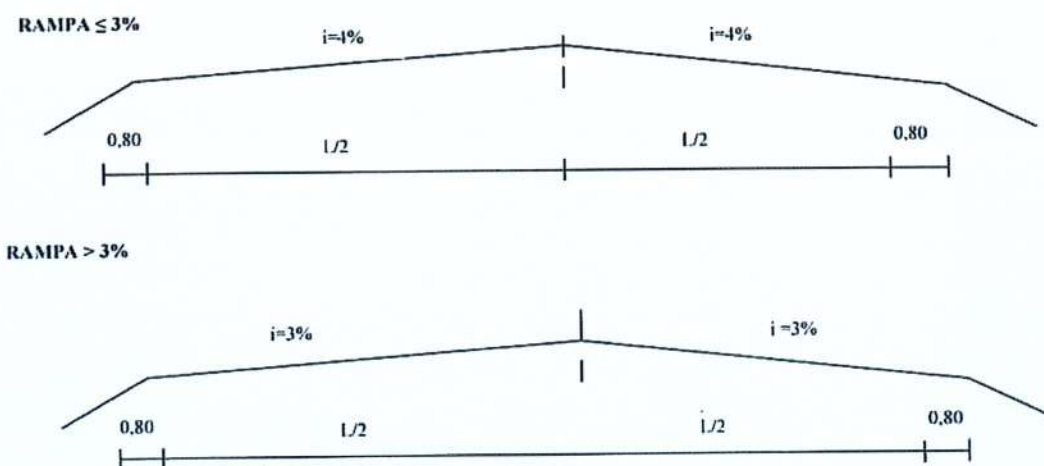
Figura 8: Inclinação transversal
