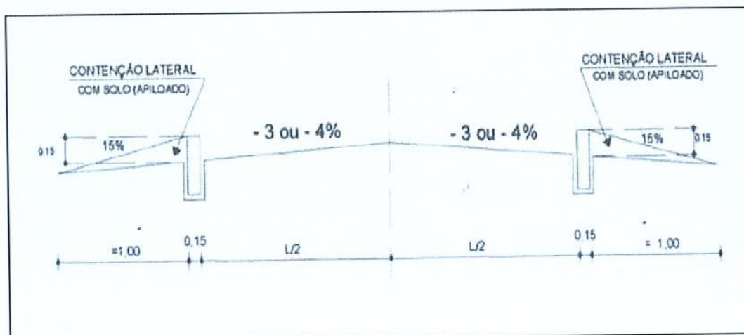
Figura 11: Contenção Lateral
